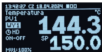
Rys.7.2.5. Ekran REGULACJA
